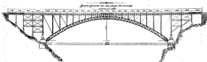
Alzado general de la estructura.
